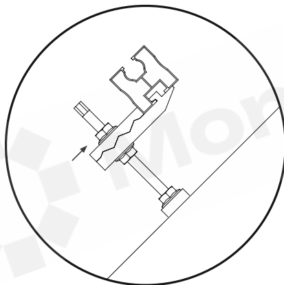
Version ① Klicktop pour vis double filetage
