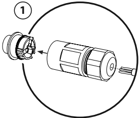
Dénuder la gaine du câble AC sur 1,5cm et enfiler le capuchon du connecteur
