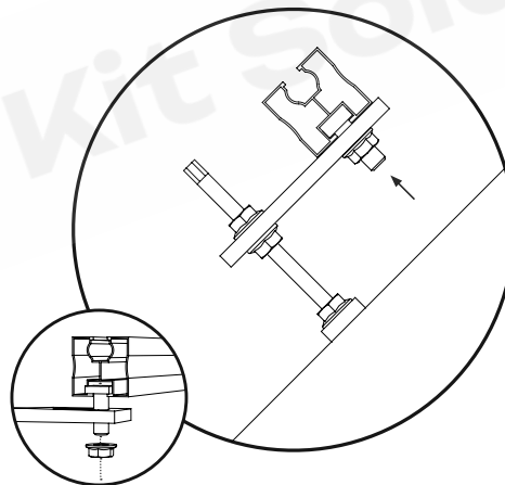
Version ② Plaque de montage avec vis à tête carré
